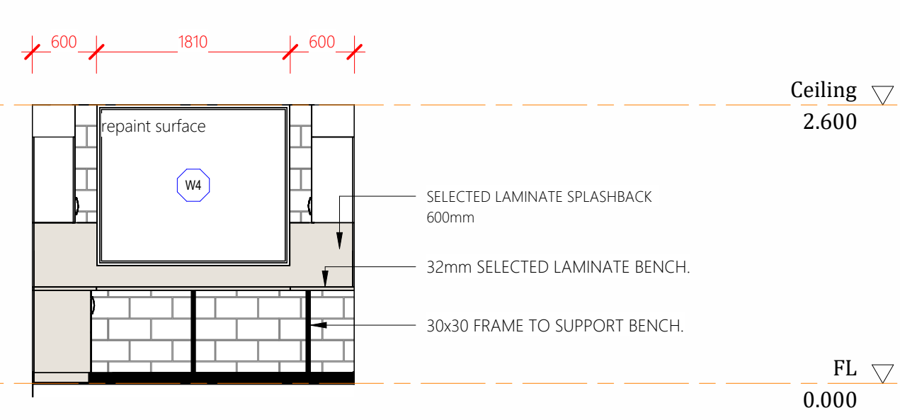
Elevation 1B
