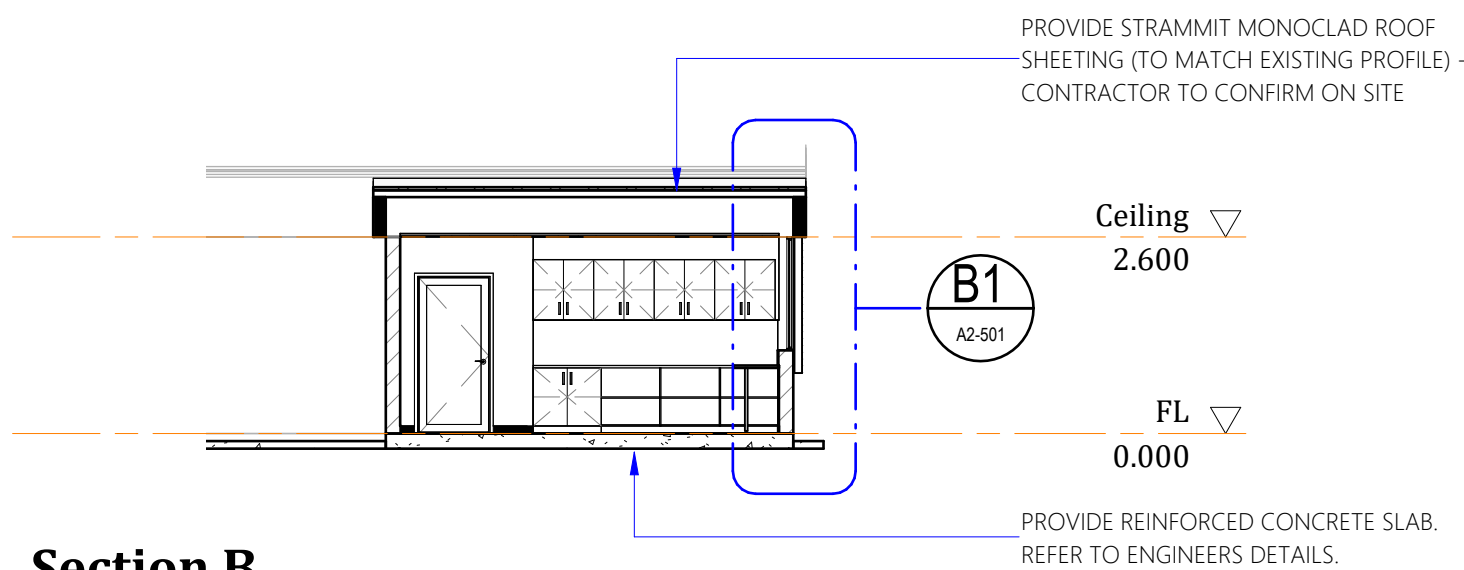
Section B 1 : 100
