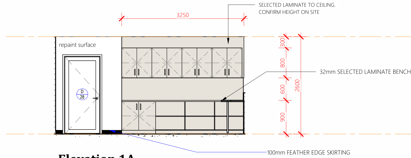
Elevation 1A
