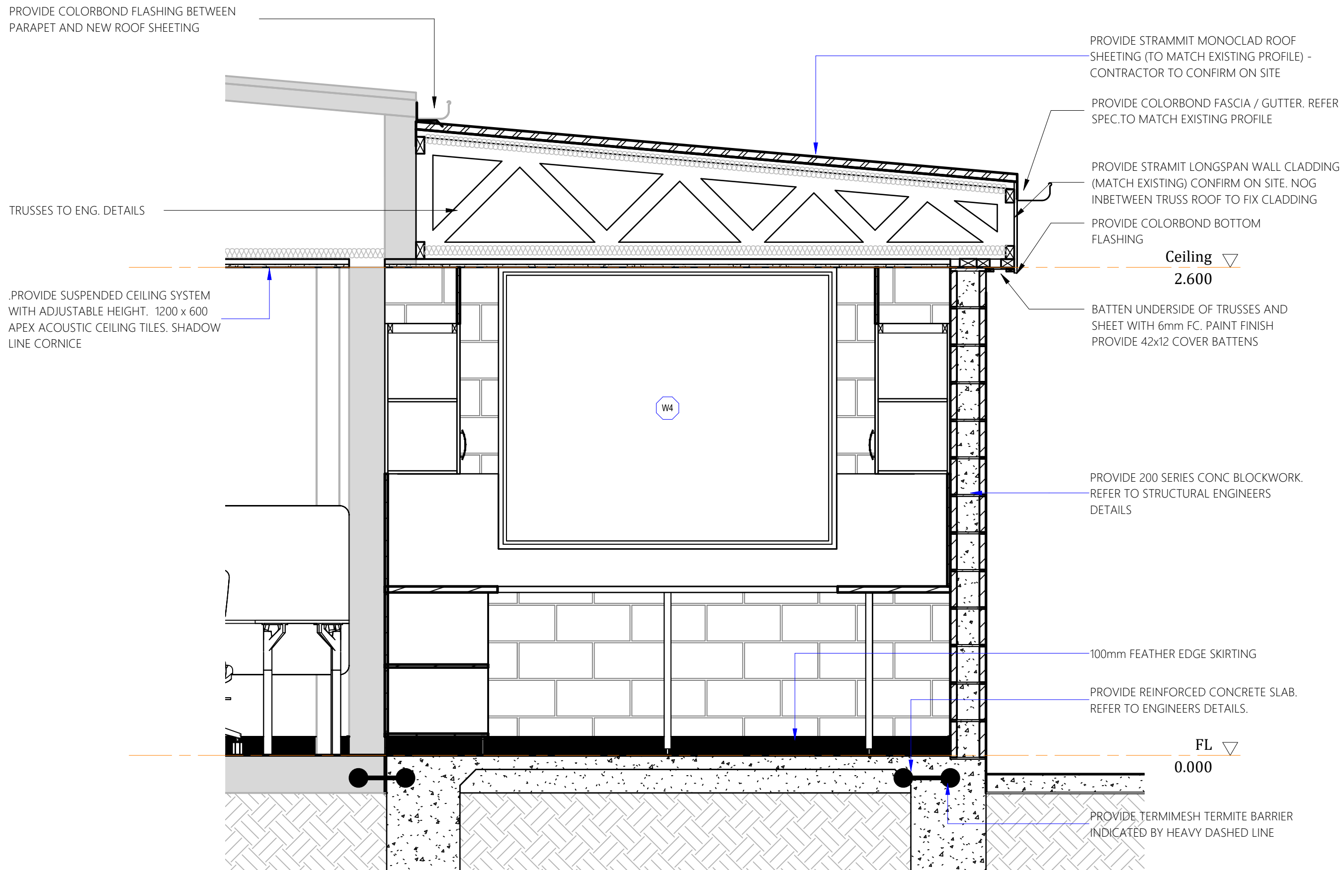
Section A1
